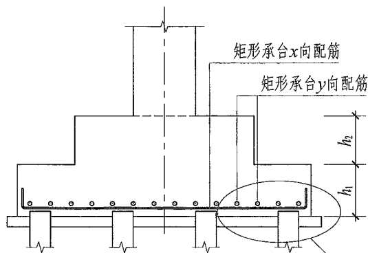
阶形截面CTj
