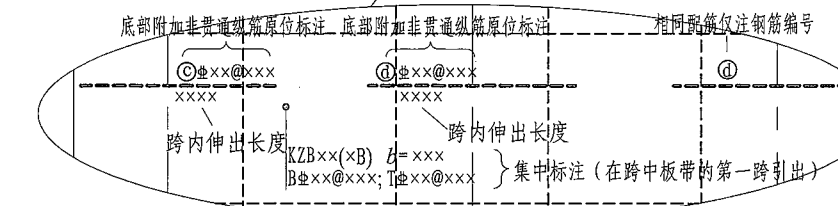
柱下板带ZXB与跨中板带KZB标注图示
