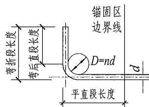
图1 90^\circ 弯折锚固示意
