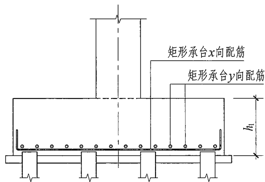
单阶形截面CTj
