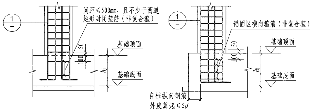
(c) 保护层厚度 > 5d ; 基础高度不满足直锚
