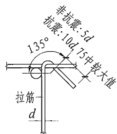
拉筋紧靠纵向钢筋并钩住箍筋
