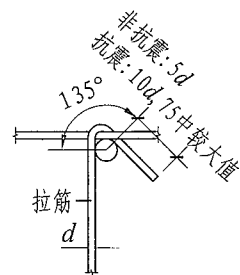
拉筋同时钩住纵筋和箍筋
