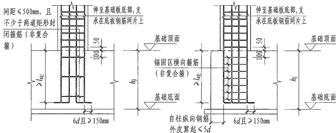
(a) 保护层厚度 > 5d ; 基础高度满足直锚
